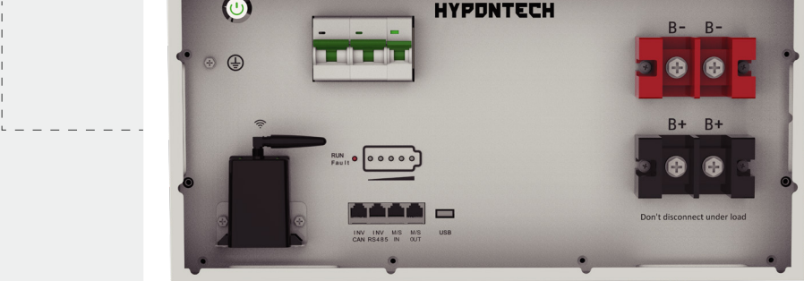
接线面板
